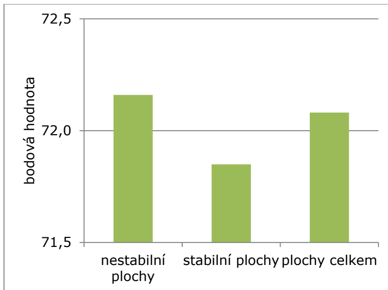
Obr. 1: Rozlohou vážená průměrná bodová hodnota produktivity půd stabilních a nestabilních ploch, pro něž byla známa bodová hodnota (70 % rozlohy území).
